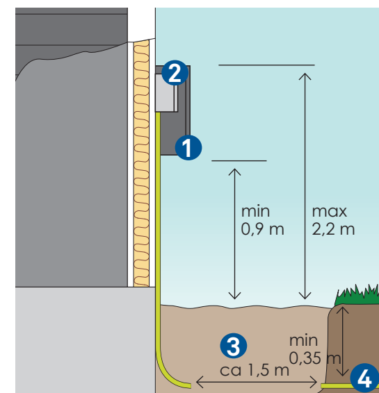
Montering av elkabel utanpå husgrund.
